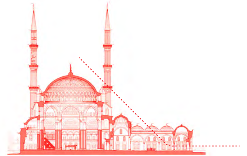
Figür 02. Edirne Selimiye Camii Uzun Kesiti
