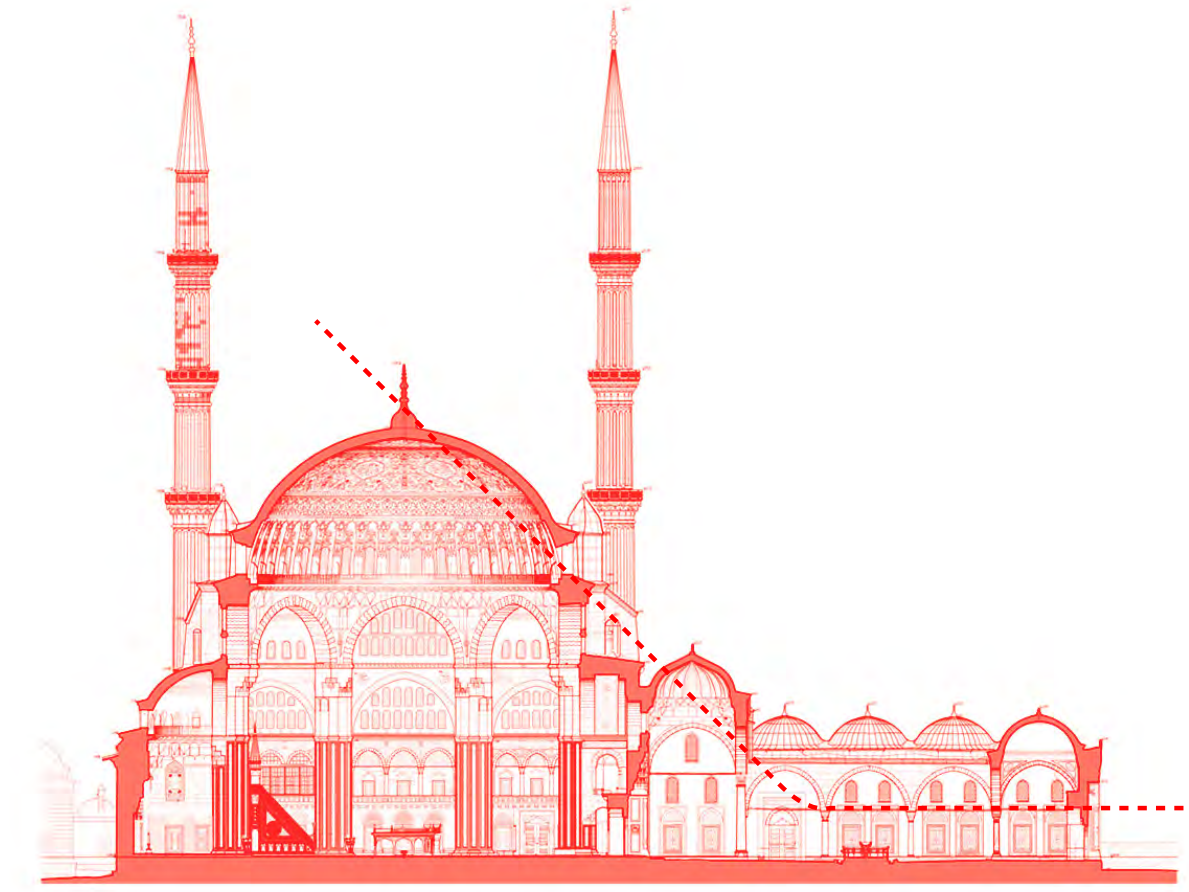
Edirne Selimiye Cami Uzun Kesiti
